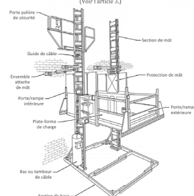
Figure 2 MCTP à mâts multiples type — Illustration des principales définitions (Voir l'article 3.)
